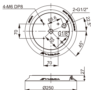
LF250-12F
