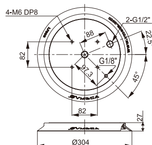
LF300-12F
