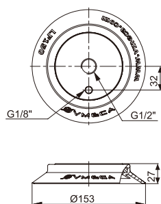
LF150-12F
